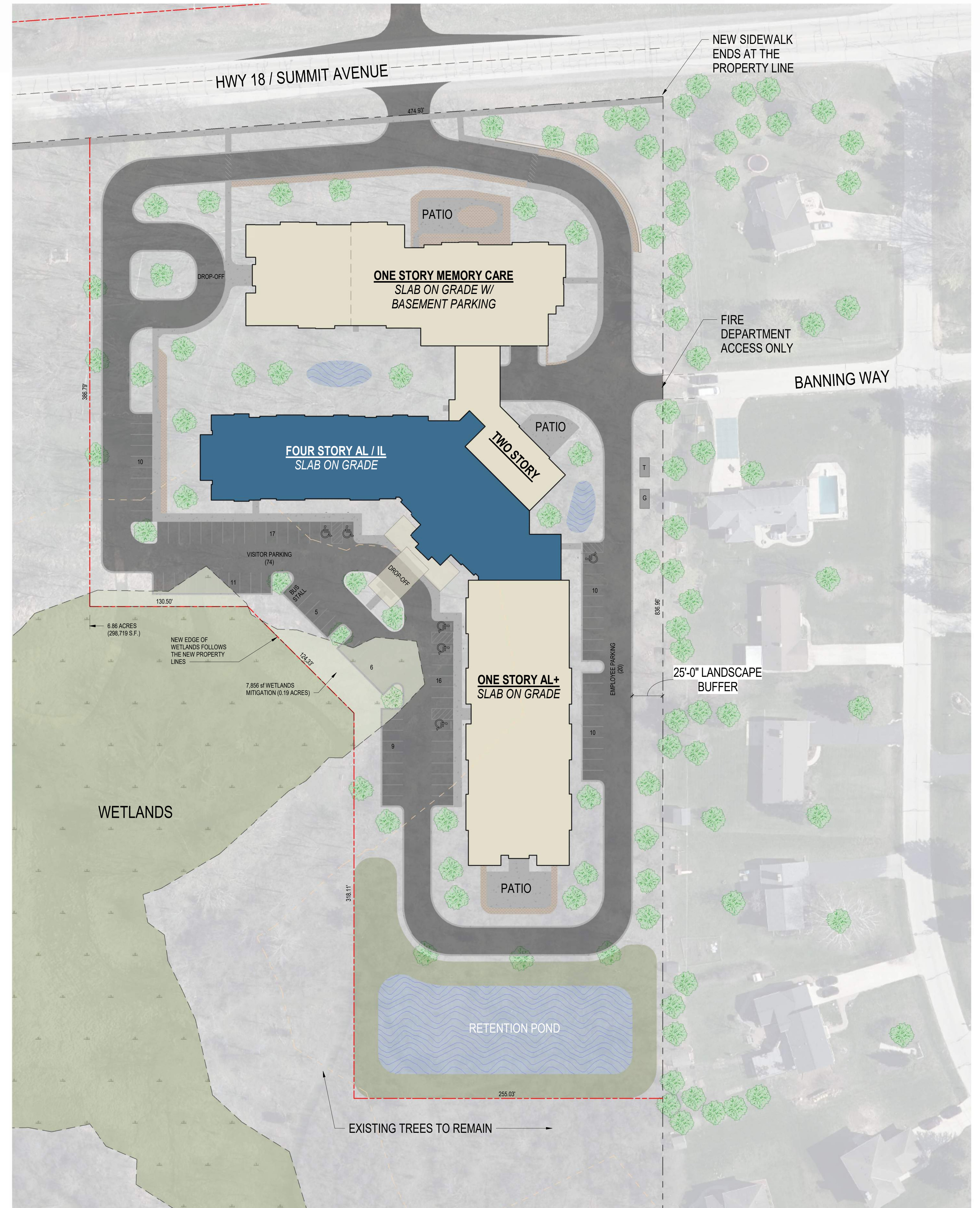
NEW SITE PLAN 11-18-2024
