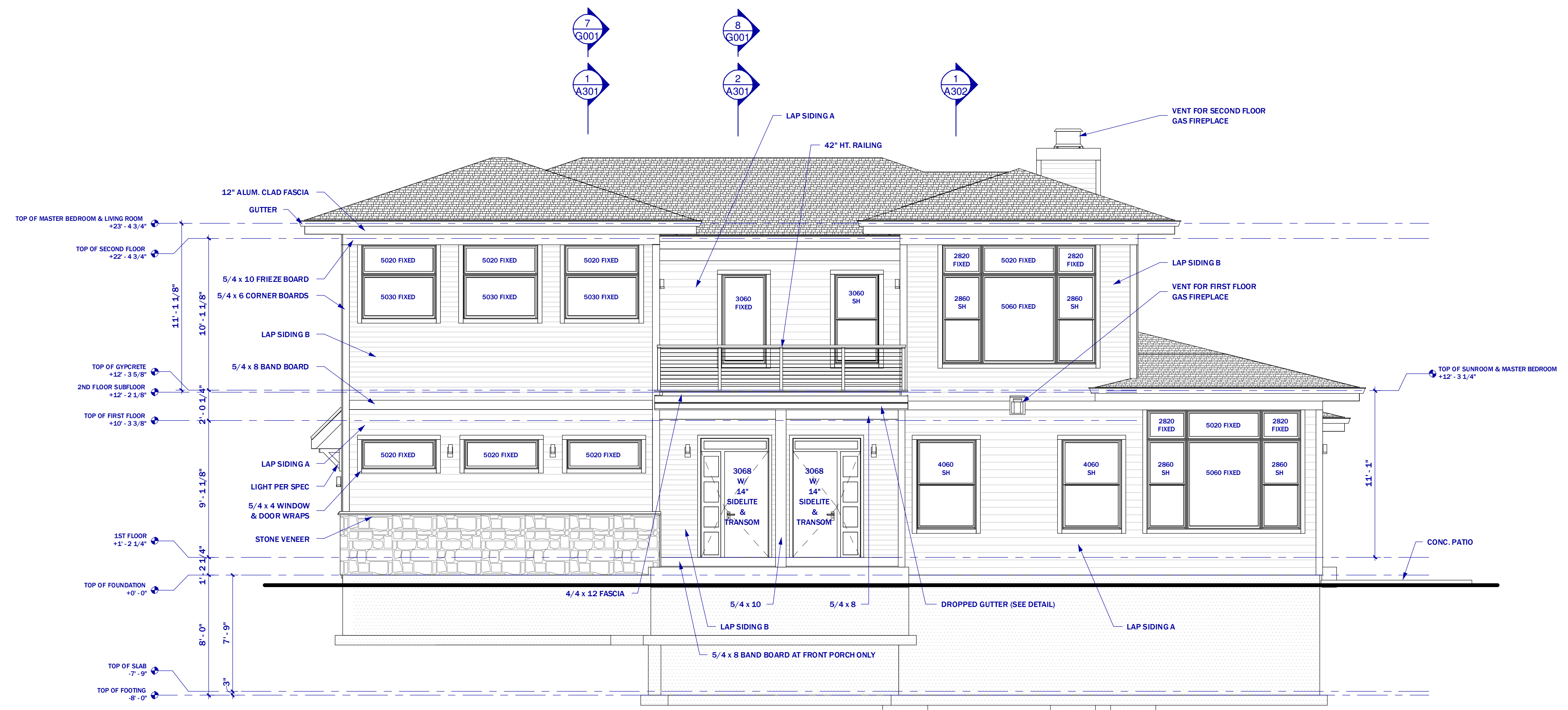
1 LEFT ELEVATION SCALE: 1/4" = 1'-0"
