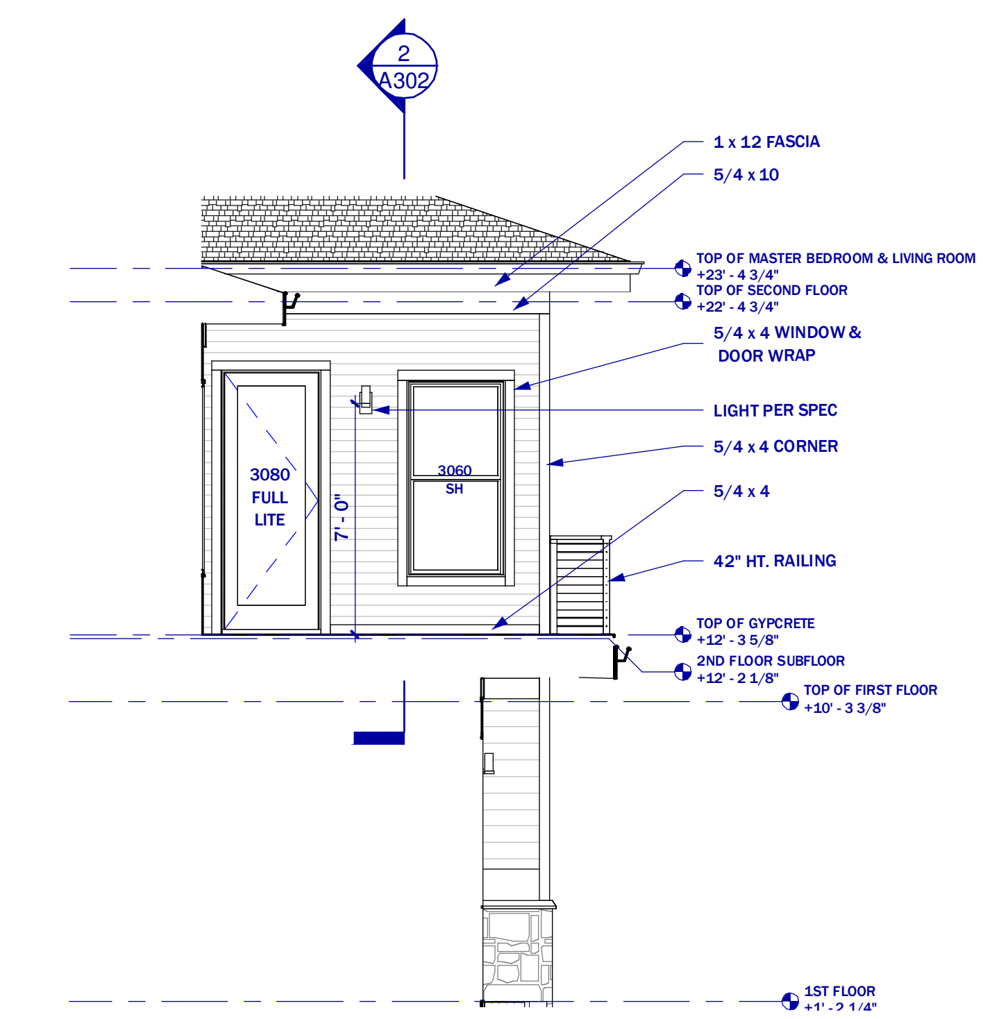
4 LEFT ELEVATION - 2 SCALE: 1/4" = 1'-0"
