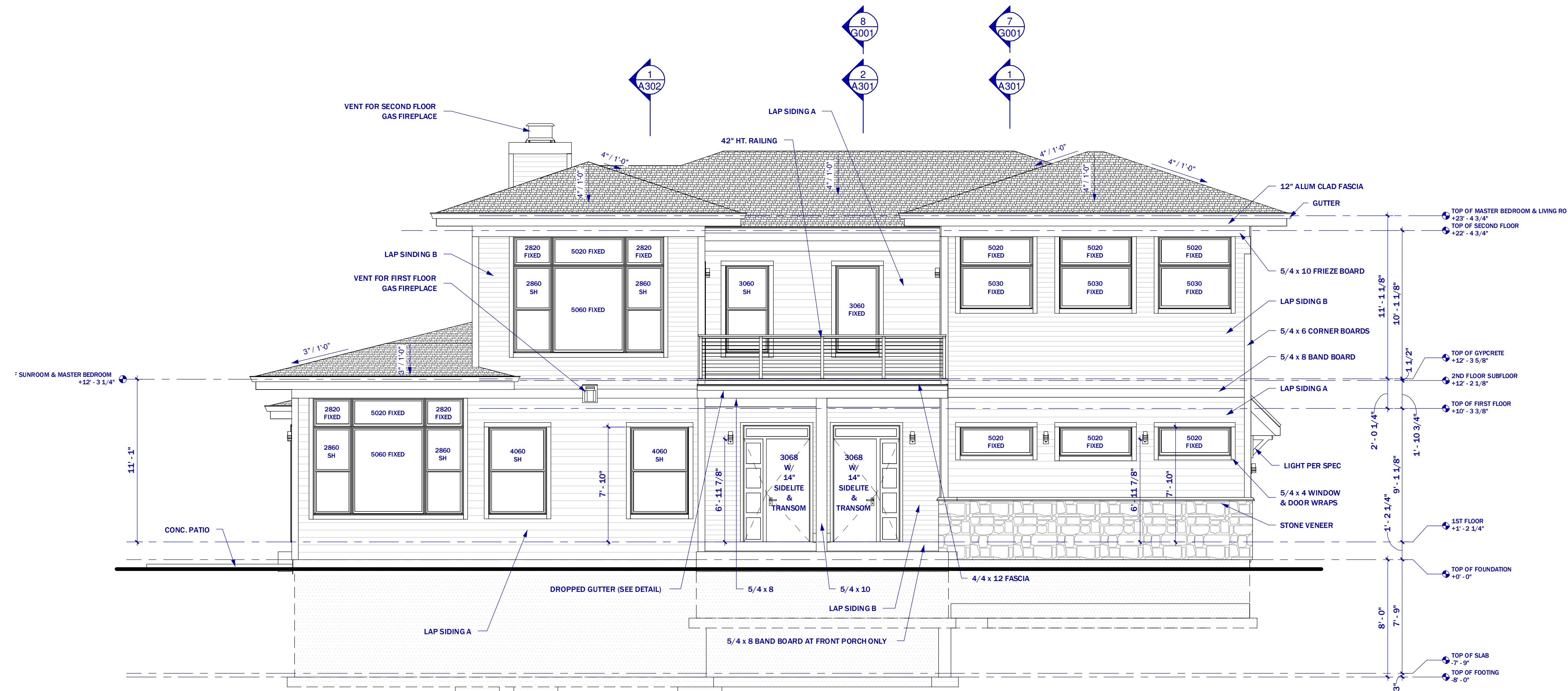
1 LEFT ELEVATION SCALE: 1/4" = 1'-0"
